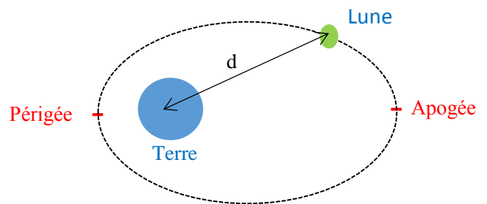
Orbite elliptique
