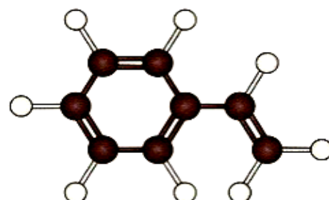
styrène
