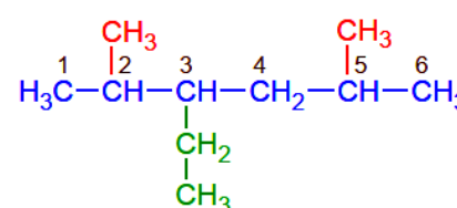
3-éthyl-2,5-diméthylhexane
