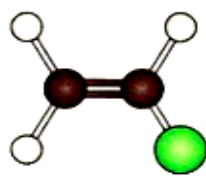
Chlorure de vinyle
