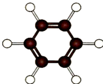
benzène
