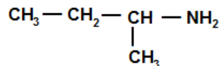
butan-2-amine
